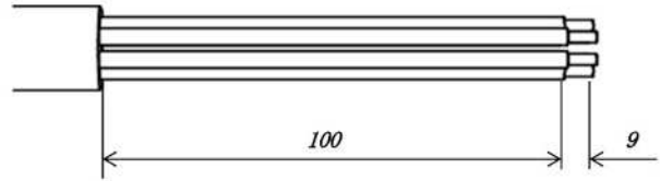
配線ケーブル推奨加工寸法
