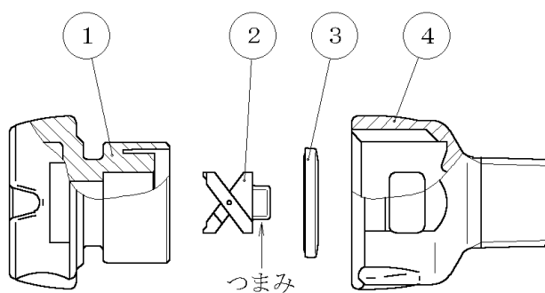
図2. 部品構成
