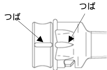
図5. 組付図
